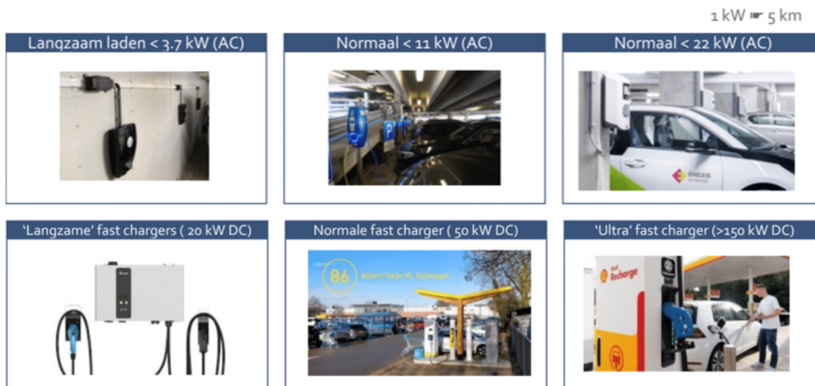
Figuur 2: Soorten laadpalen en bijbehorende vermogens
