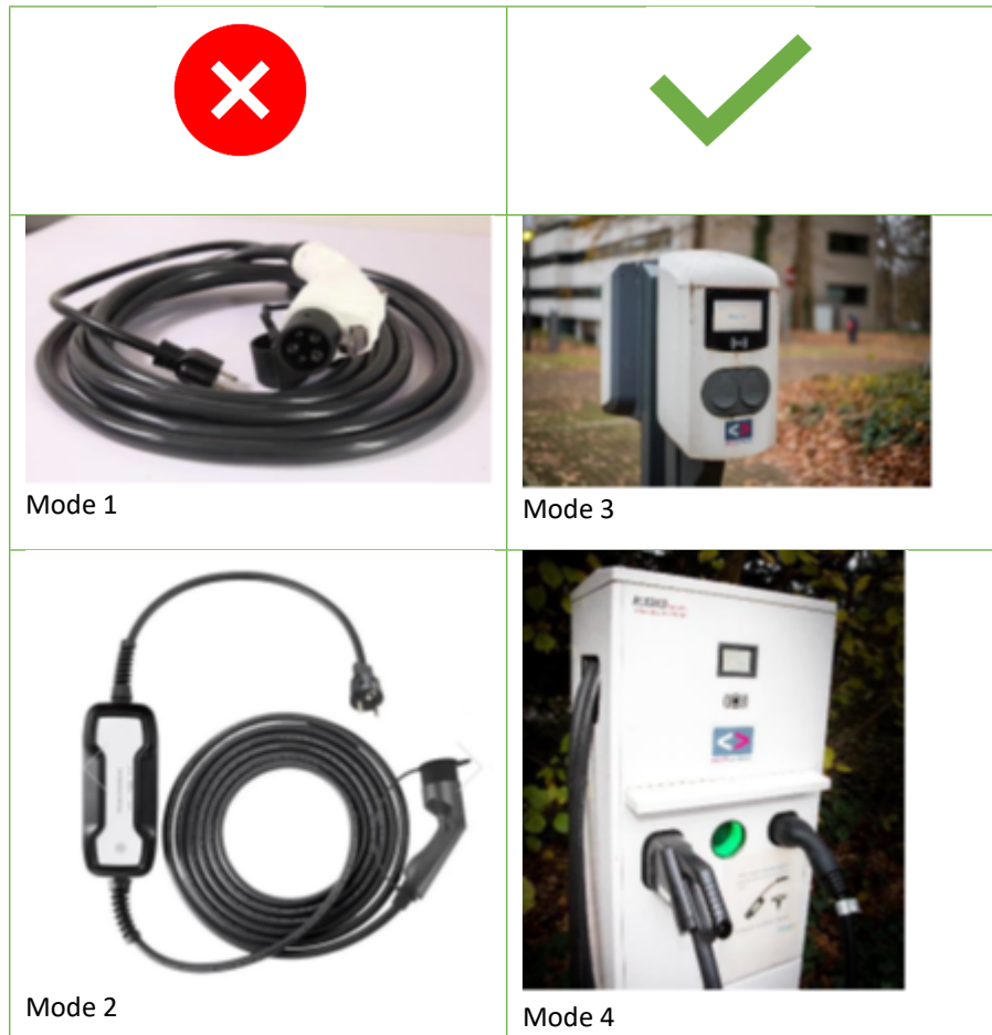
Figuur 8: Minder veilige modes van laden (mode 1 en 2) en veiligere modes van laden (mode 3 en 4)
